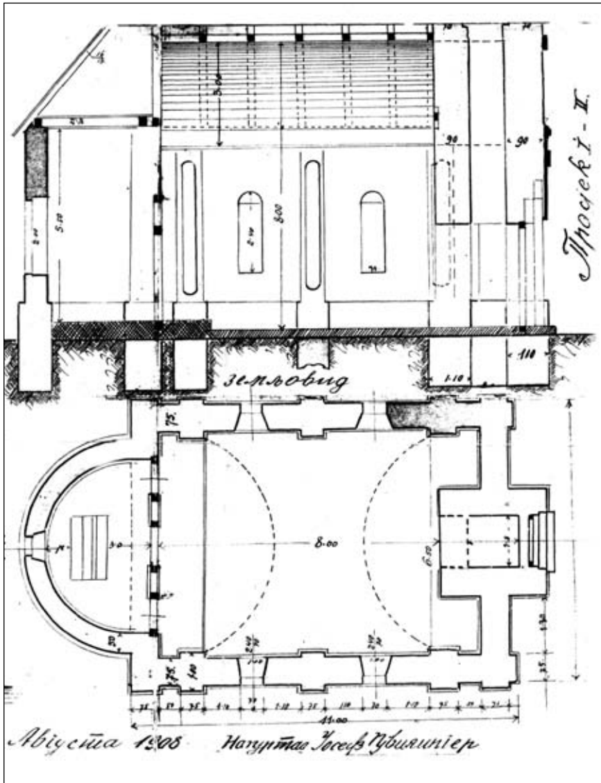
Основа и подужни пресек цркве, из плана Јозефа Цвилингера
