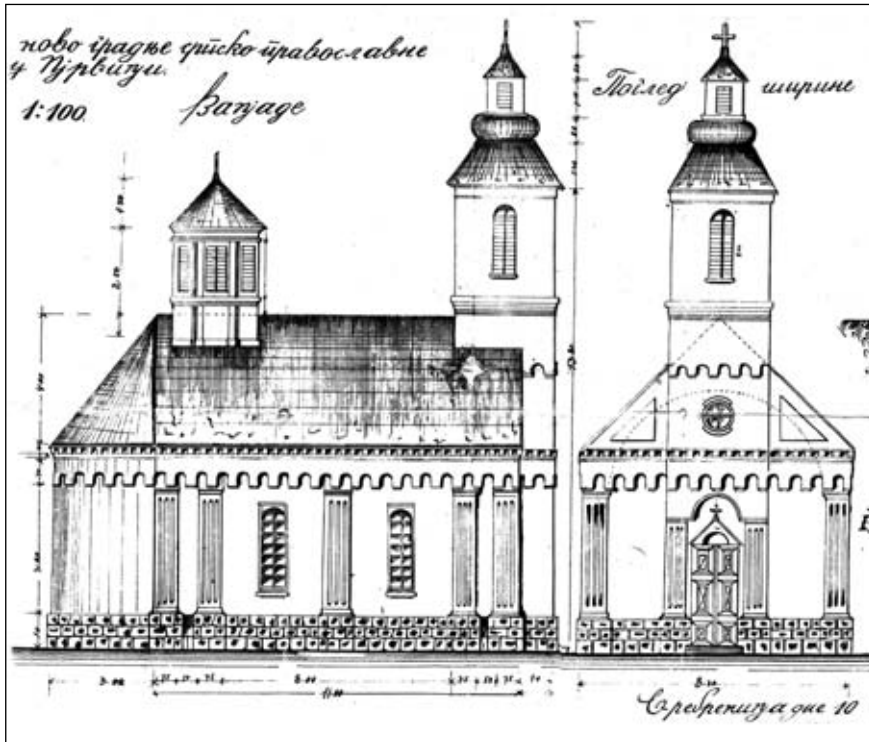
Фасада цркве, детаљ из плана Јозефа Цвилингера
