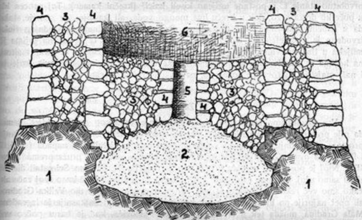
Sl. 12. Grad Borač: vertikalni presjek temelja kule s cisternom (šematični prikaz); 1 prirodna stijena, 2 pjesak, odnosno šupljina cisterne, 3 kaša lomljenog kamena i maltera, 4 oplata zidova, 5 rupa kroz koju se uzimala voda, 6 podrumski prostor nad cisternom.
